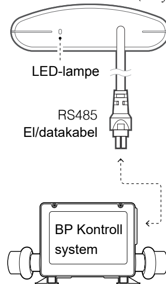
GATEWAY ULTRA-enheden (vist fra siden)
