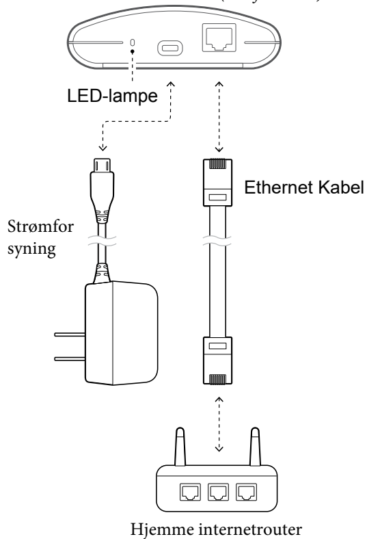
GATEWAY ULTRA-enheden (vist fra siden)
